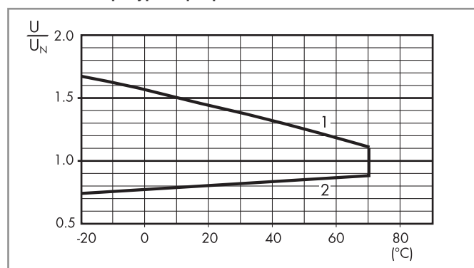
R 41- Отношение рабочего диапазона для AC к температуре окр. среды
